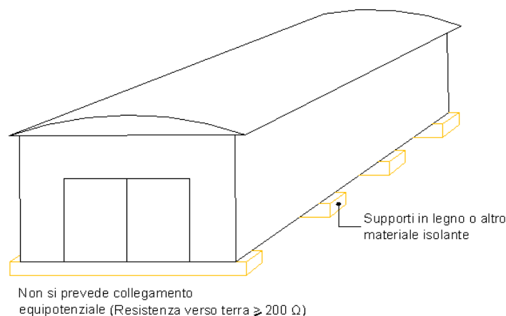
Figura 1 – Baracca metallica isolata
